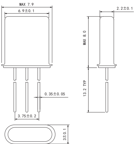
THREE LEADS (三引线) UNIT (单位): mm (毫米)
