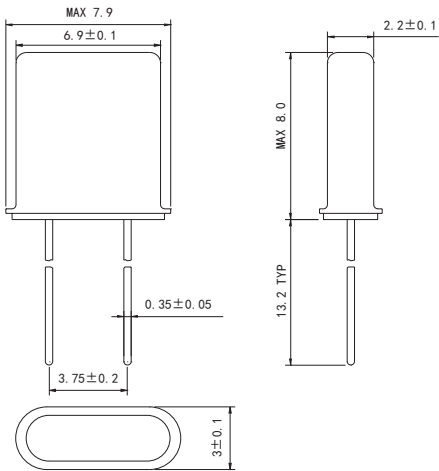
TWO LEADS (两引线) UNIT (单位): mm (毫米)
